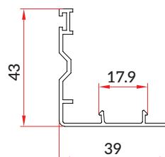
Sliding Door Interlock (SD-GF-050)
