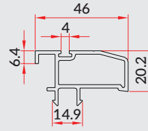
Door Sash Cover (SCW-GF-N108)
