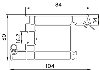
Inward Door Sash (CW-GF-046)
