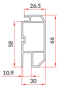
Sliding Door Mesh Sash (SD-GF-002)
