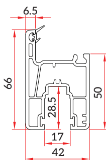
Sliding Door Sash (SW-GF-031)
