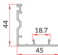
Sliding Door Interlock (SW-GF-026)
