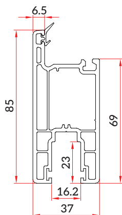
Sliding Door Sash (SW-GF-033)
