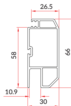
Sliding Door Mesh Sash (SD-GF-002)
