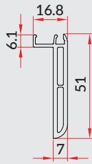
Universal Cornice (SCW-GF-N106)
