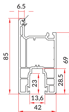
Sliding Mega Door Sash (SD-GF-001)
