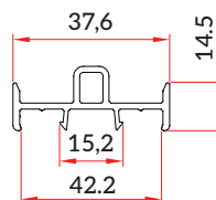
Sash Connector (SW-GF-029)
