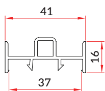
Sash Connector (SW-GF-015)
